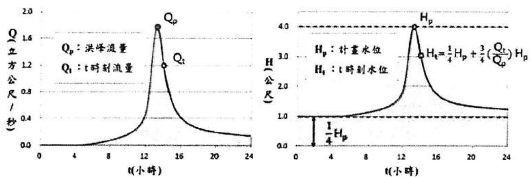
附圖 1 SCS 無因次單位歷線示意圖
