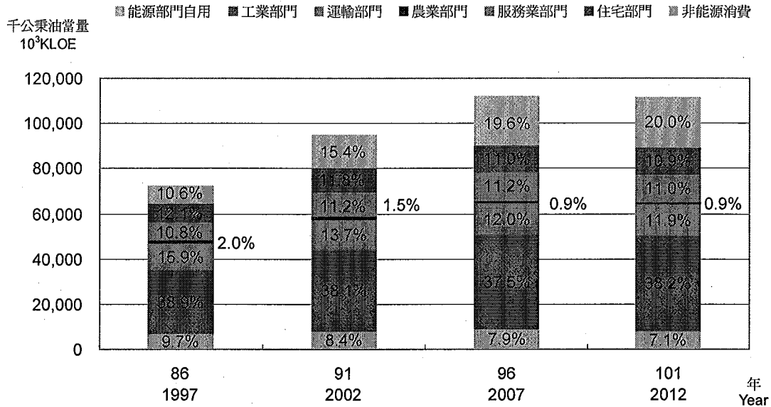
圖 2 我國部門能源消費趨勢圖
